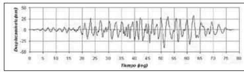
Figura 47: Registro Sismo Frontal. Registro de desplazamiento en función del tiempo.
