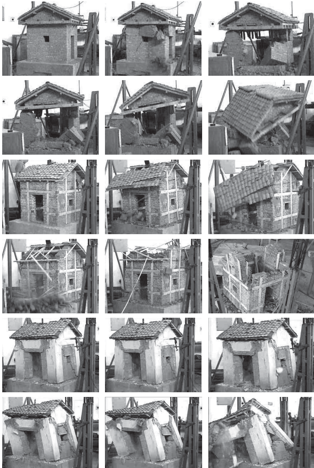
Figuras 48 a 51: Mecanismo de colapso de vivienda de adobe sin ningún refuerzo.
