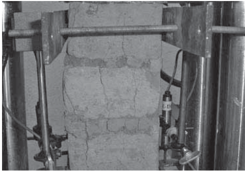
Figura 27: Ensayo de compresión de adobe.
