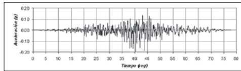
Figura 46: Registro Sismo Frontal. Registro de aceleración en función del tiempo.
