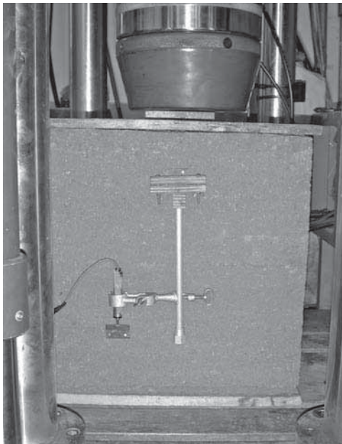
Figura 30: Ensayo de tracción diagonal.
